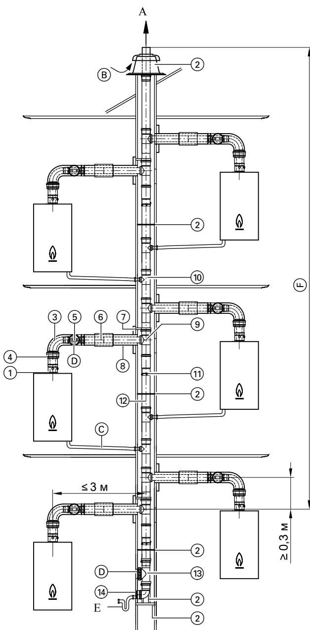
2 водогрейных котла на этаж
