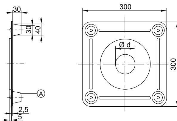
А Распорка
