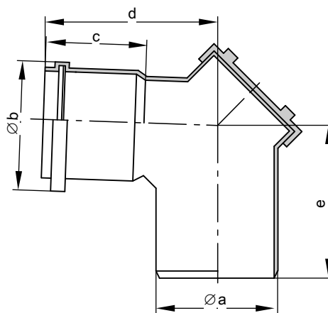
Ревизионное колено
